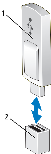
図 3-18 USB メモリキーの取り外しまたは取り付け
