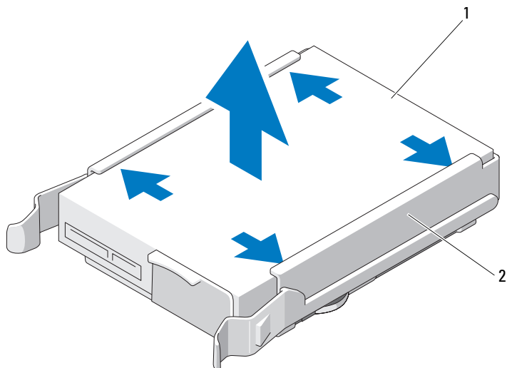
図 3-10 ハードドライブをハードドライブブラケットから取り外す方法
