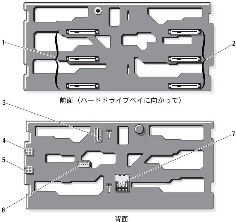
図 6-2 SAS バックプレーンボードコネクタ
