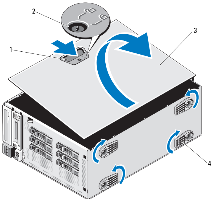
図 3-5 システムカバーの開閉
