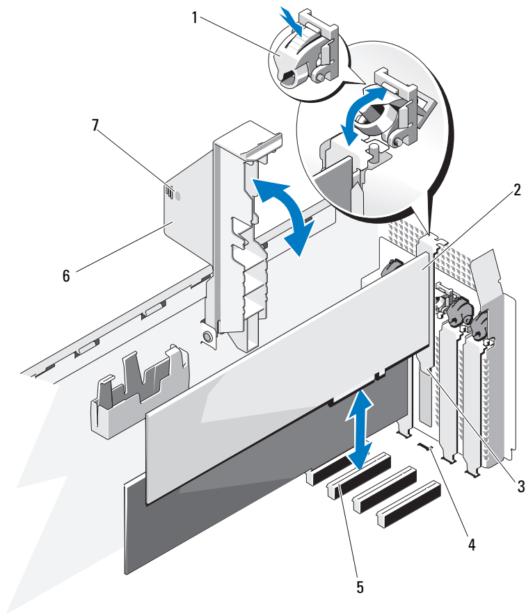
図 3-14 拡張カードの取り外しと取り付け
