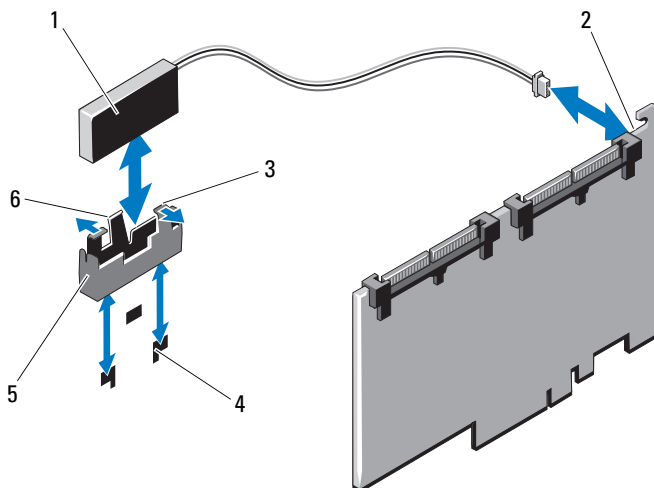
図 3-15 RAID バッテリーの取り付けと取り外し
