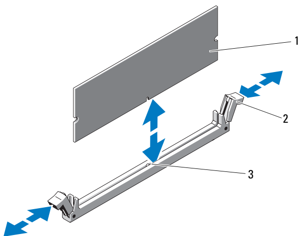
図 3-13 メモリモジュールの取り付けと取り外し
