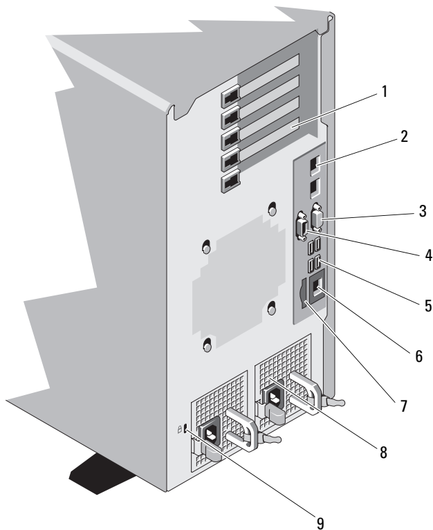
図 1-4 背面パネルの機能およびインジケータ
