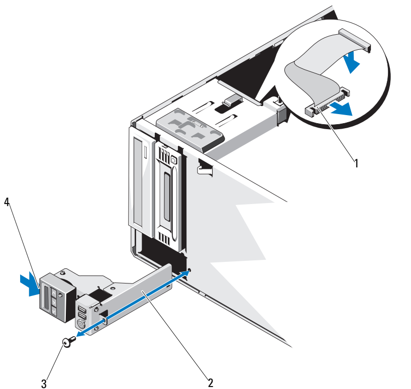
図 3-26 コントロールパネルの取り外しと取り付け
