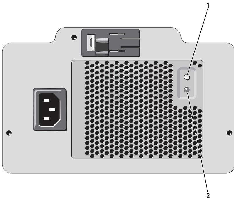
図 1-7 非冗長電源ユニットのステータスインジケータ
