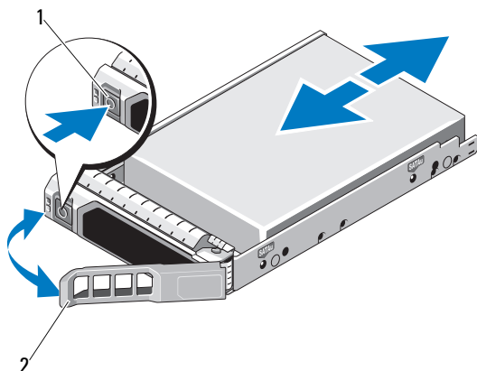
図 3-7 ホットスワップ対応ハードドライブの取り外しと取り付け
