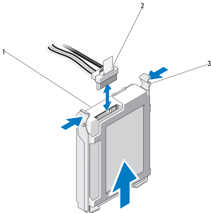
図 3-9 ケーブル接続されたハードドライブの取り外しと取り付け
