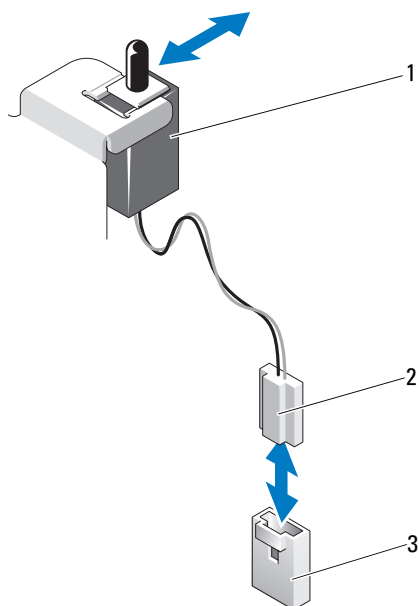
図 3-25 シャーシイントルージョンスイッチの取り外しと取り付け
