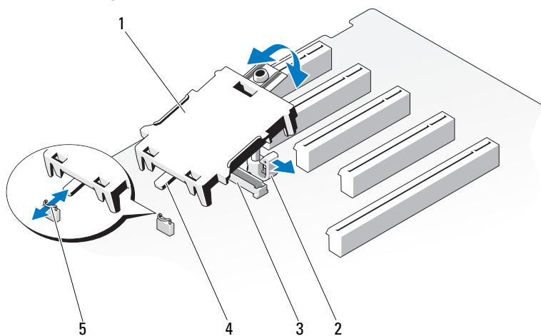
図 3-19 iDRAC6 Express カードの取り外しと取り付け
