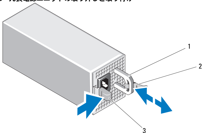
図 3-16 冗長電源ユニットの取り外しと取り付け
