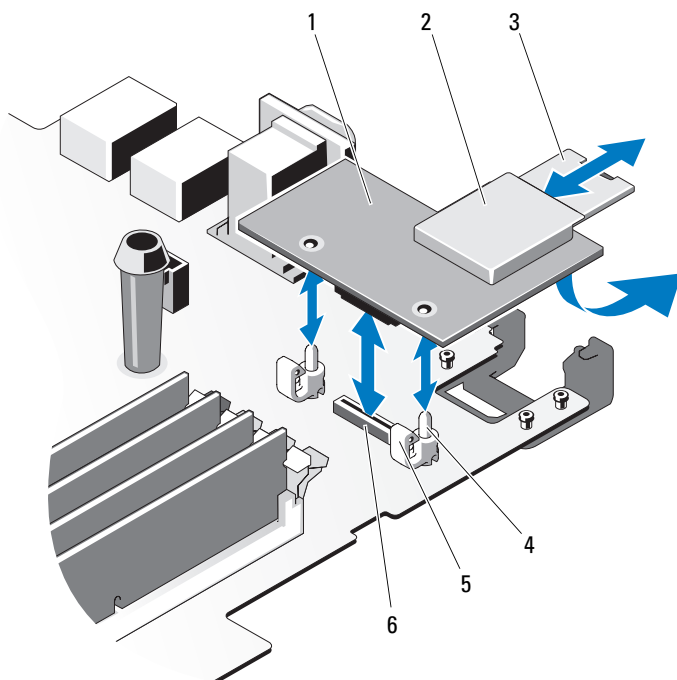
図 3-20 iDRAC6 Enterprise カードの取り外しと取り付け
