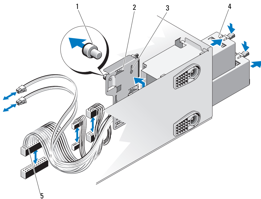
図 3-28 配電基板の取り外しと取り付け
