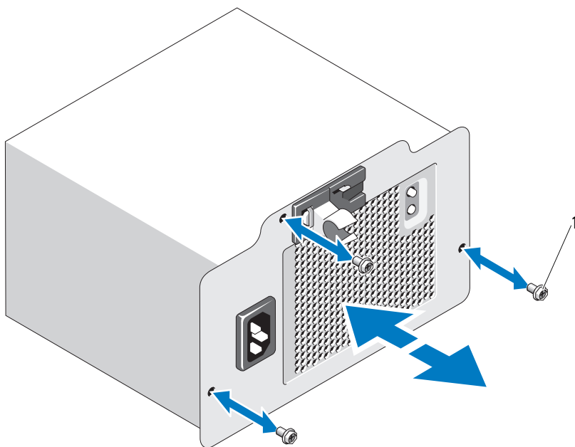
図 3-17 非冗長電源ユニットの取り外しと取り付け
