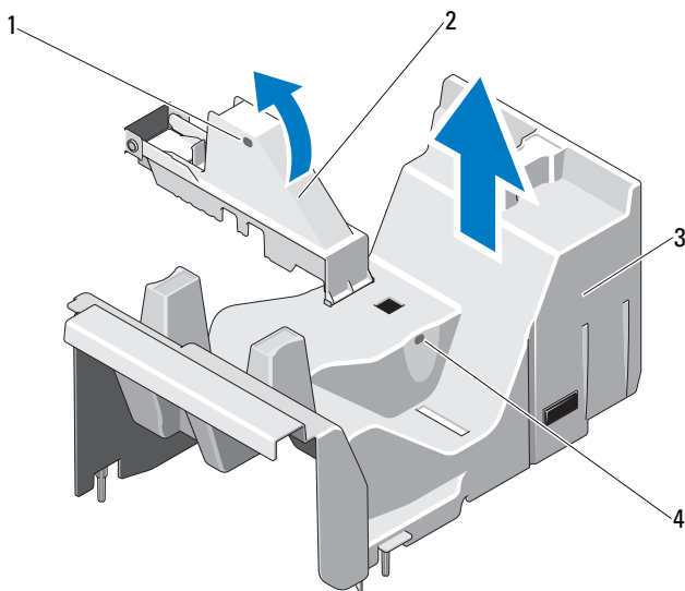
図 3-6 エアフローカバーの取り外しと取り付け
