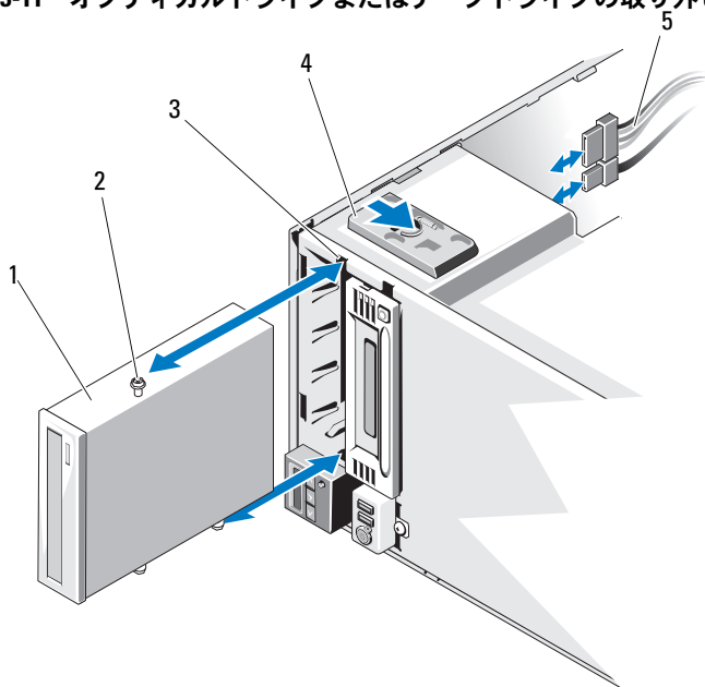
図 3-11 オプティカルドライブまたはテープドライブの取り外しと取り付け
