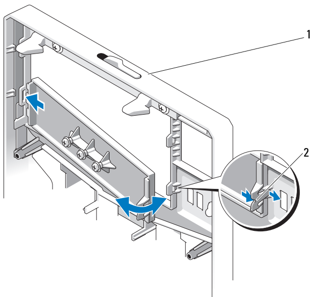
図 3-3 前面ベゼルカバーの取り外しと取り付け
