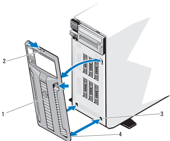
図 3-2 前面ベゼルの取り外しと取り付け
