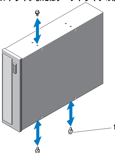
図 3-12 光学ドライブまたはテープドライブの肩付きネジの取り付け
