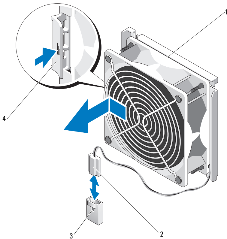
図 3-21 システムファンの取り外しと取り付け
