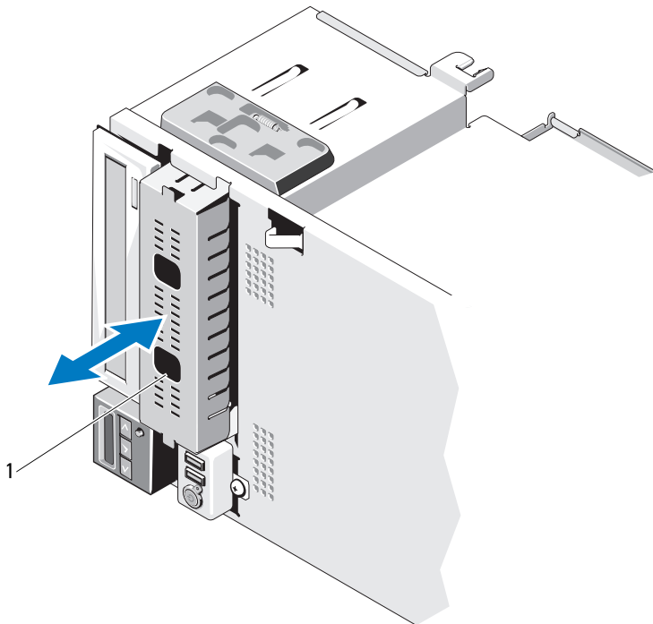
図 3-4 EMI フィラーの取り外しと取り付け
