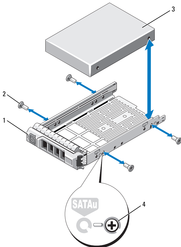
図 3-8 ハードドライブをドライブキャリアに取り付ける方法
