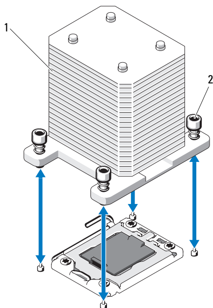
図 3-22 ヒートシンクの取り付けと取り外し
